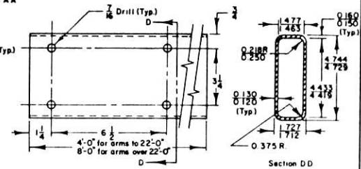
SLEEVE Aluminum 6061-T6
