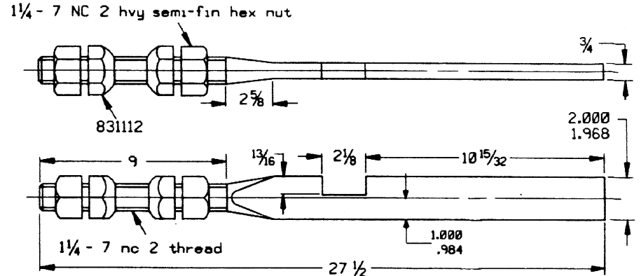
831113 LOCK ROD - R. OR L. HAND T-20
